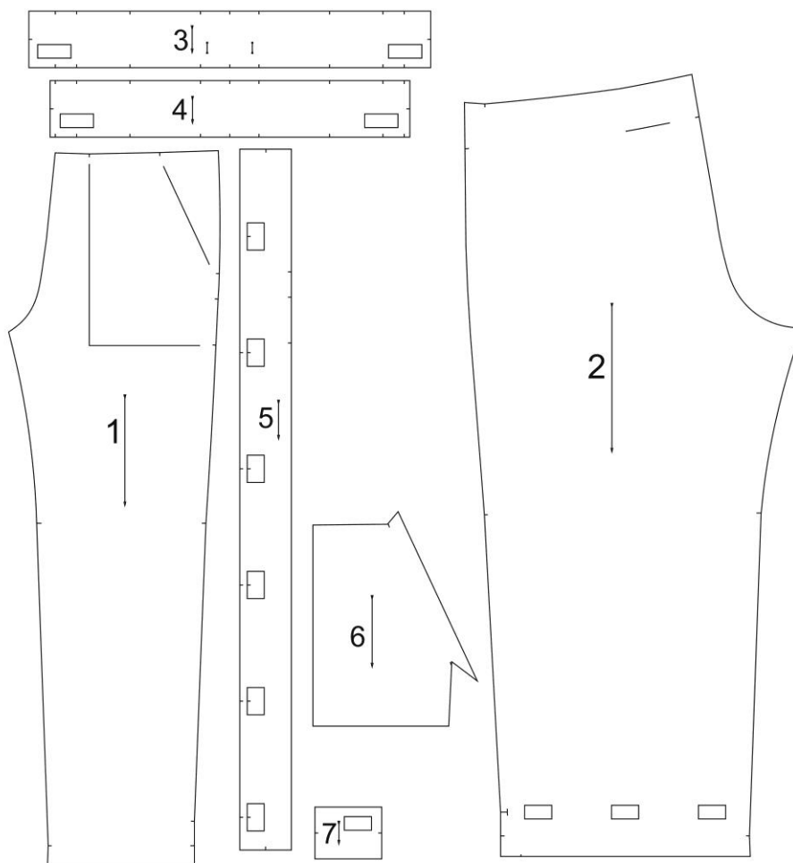
Рисунок Д2 – Орієнтовний зовнішній вигляд деталей предмета
