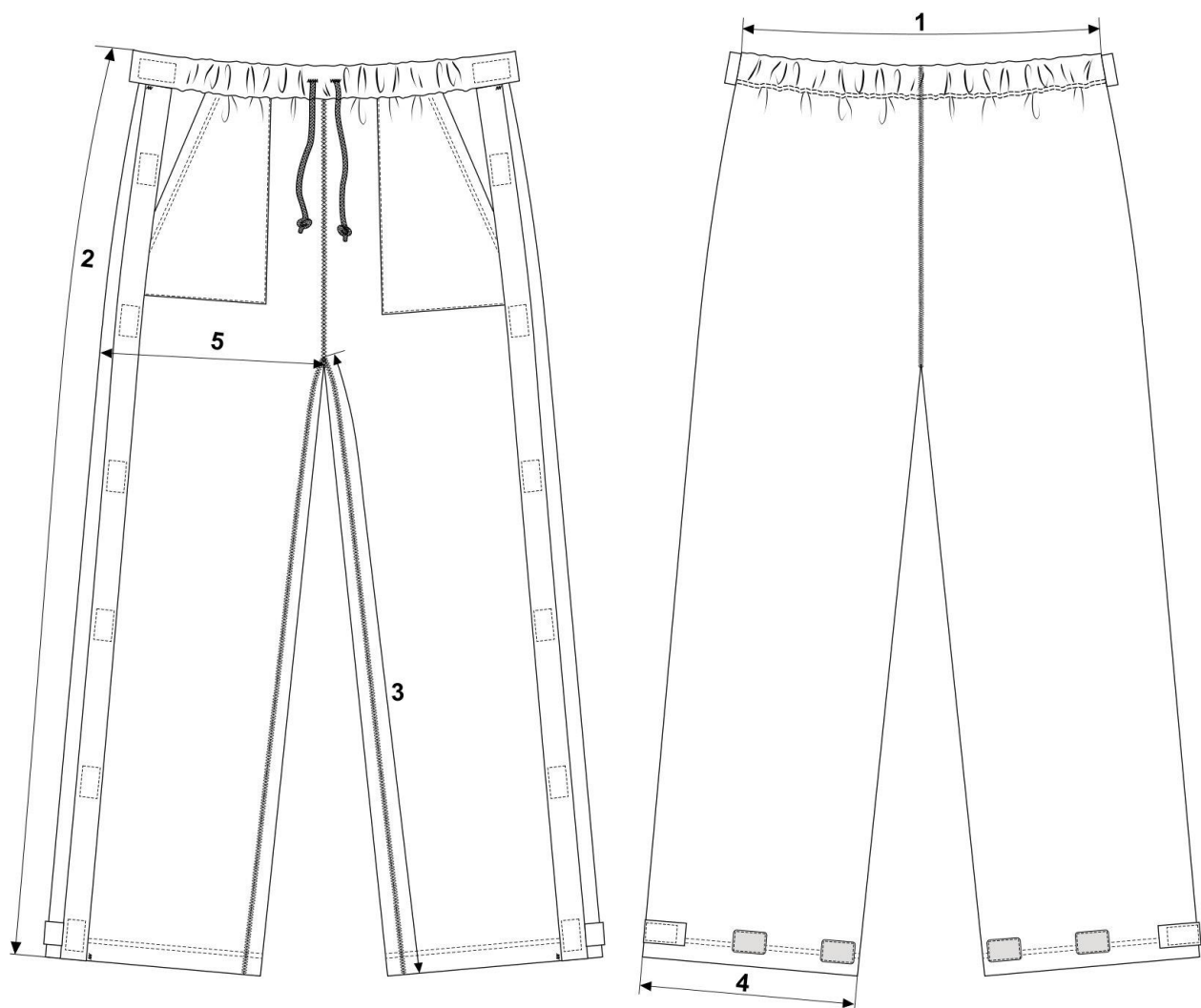
Рисунок Д1 – Орієнтовний зовнішній вигляд предмета та позначення лінійних вимірів (вид спереду та ззаду)
