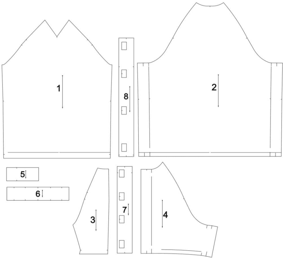
Рисунок Д2 – Орієнтовний зовнішній вигляд деталей предмета
