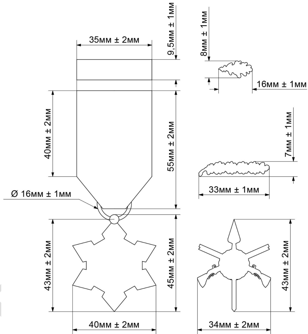
Рисунок 2 – Лінійні розміри предмета
