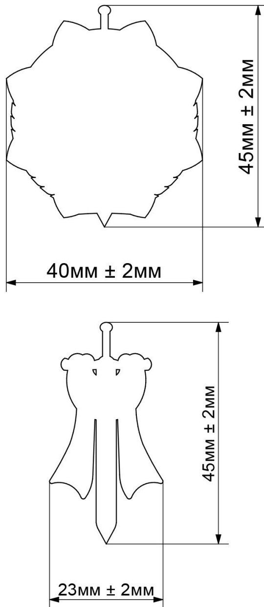
Рисунок 2 – Лінійні розміри предмета
