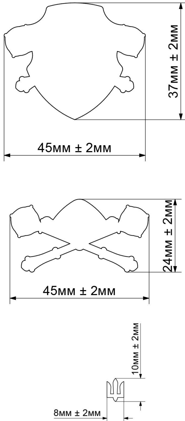
Рисунок 2 Лінійні розміри предмета
