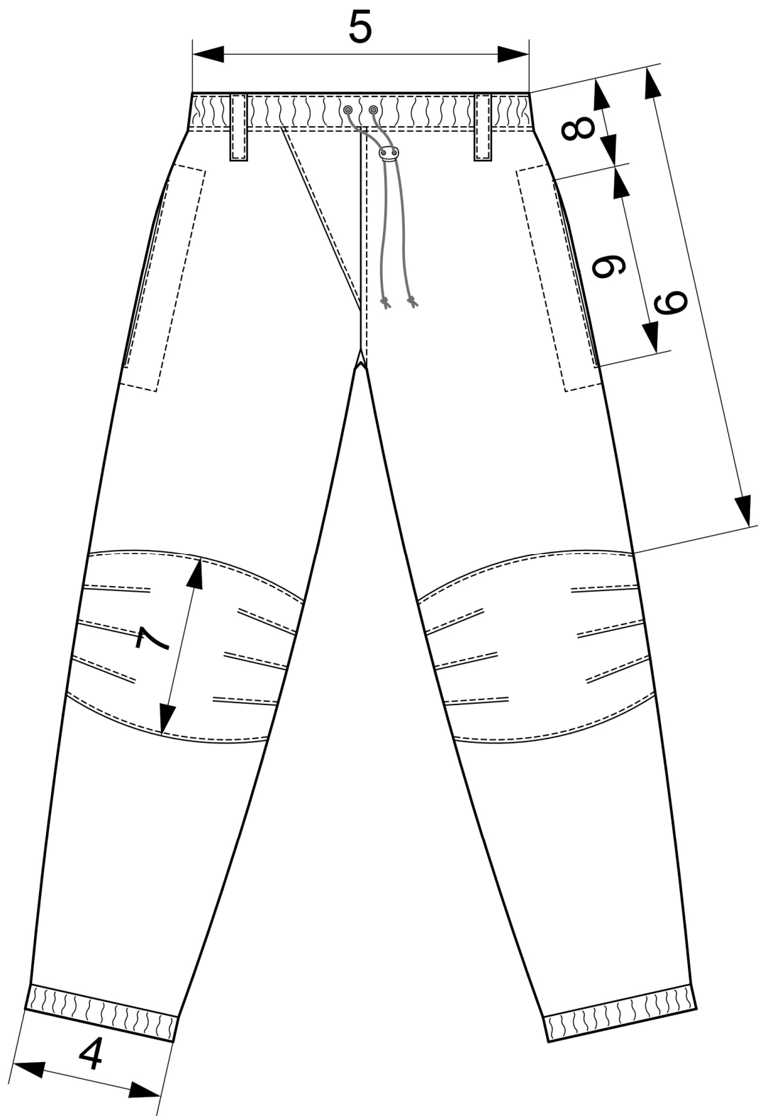
Рисунок Д2.4 – Орієнтовні позначення лінійних вимірів предмета 2 (вигляд спереду)
