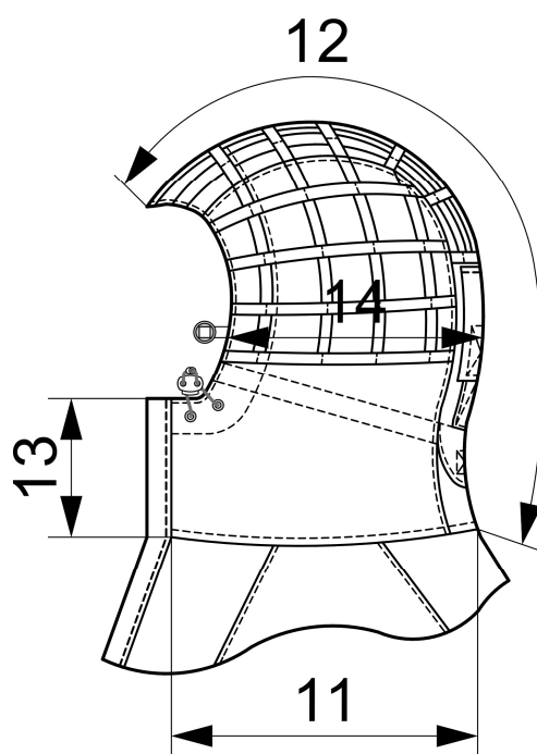
Рисунок Д2.3 – Орієнтовні позначення лінійних вимірів капюшона предмета 1 (вигляд збоку)
