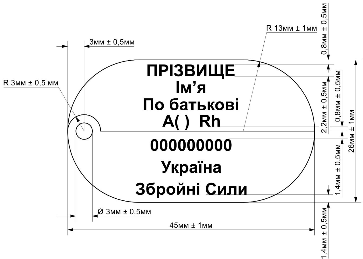
Рисунок 5 Лінійні розміри предмета
