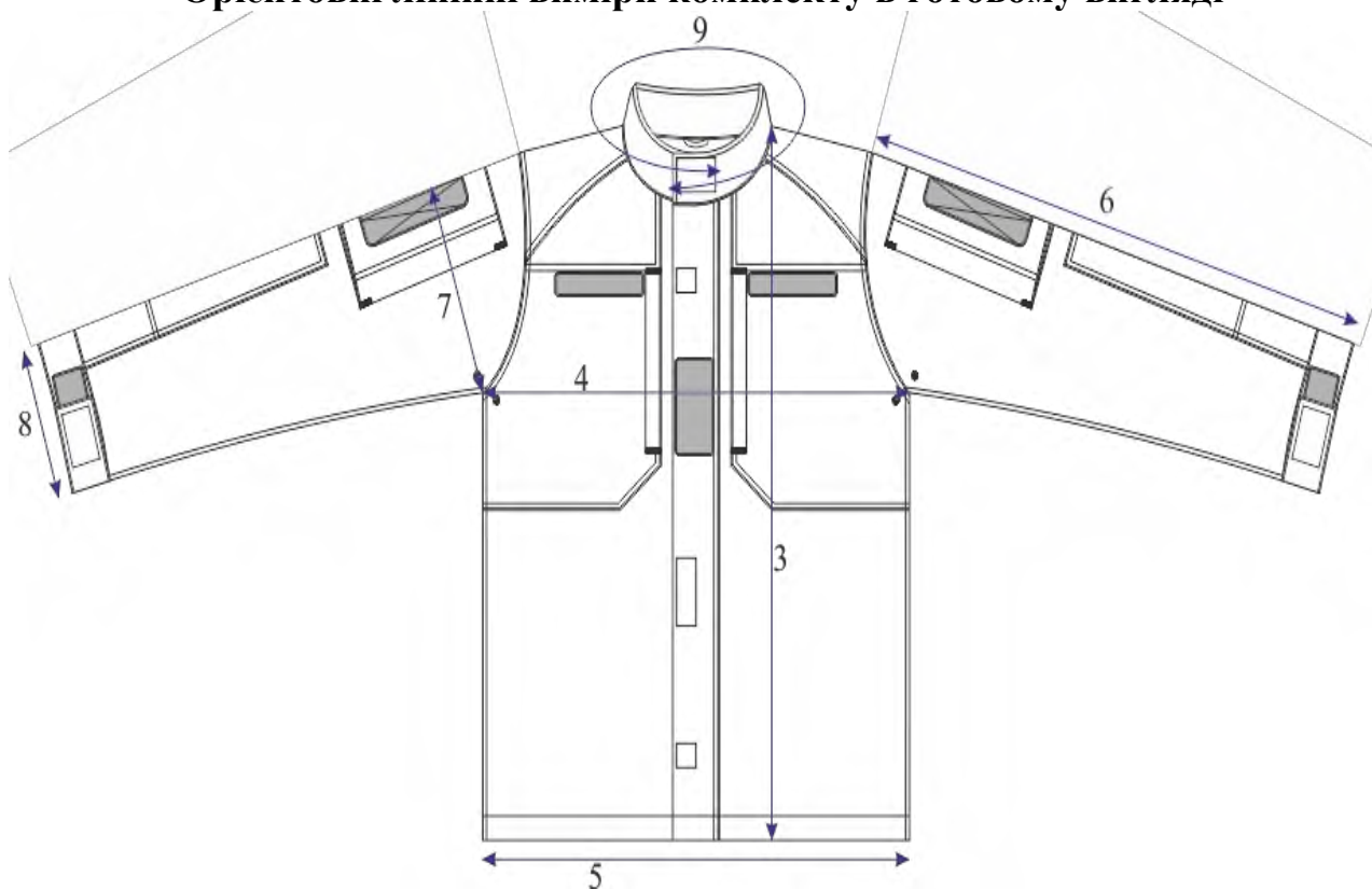
Рисунок ДЗ.1. – Позначення лінійних вимірів предмета 1 (вид спереду)
