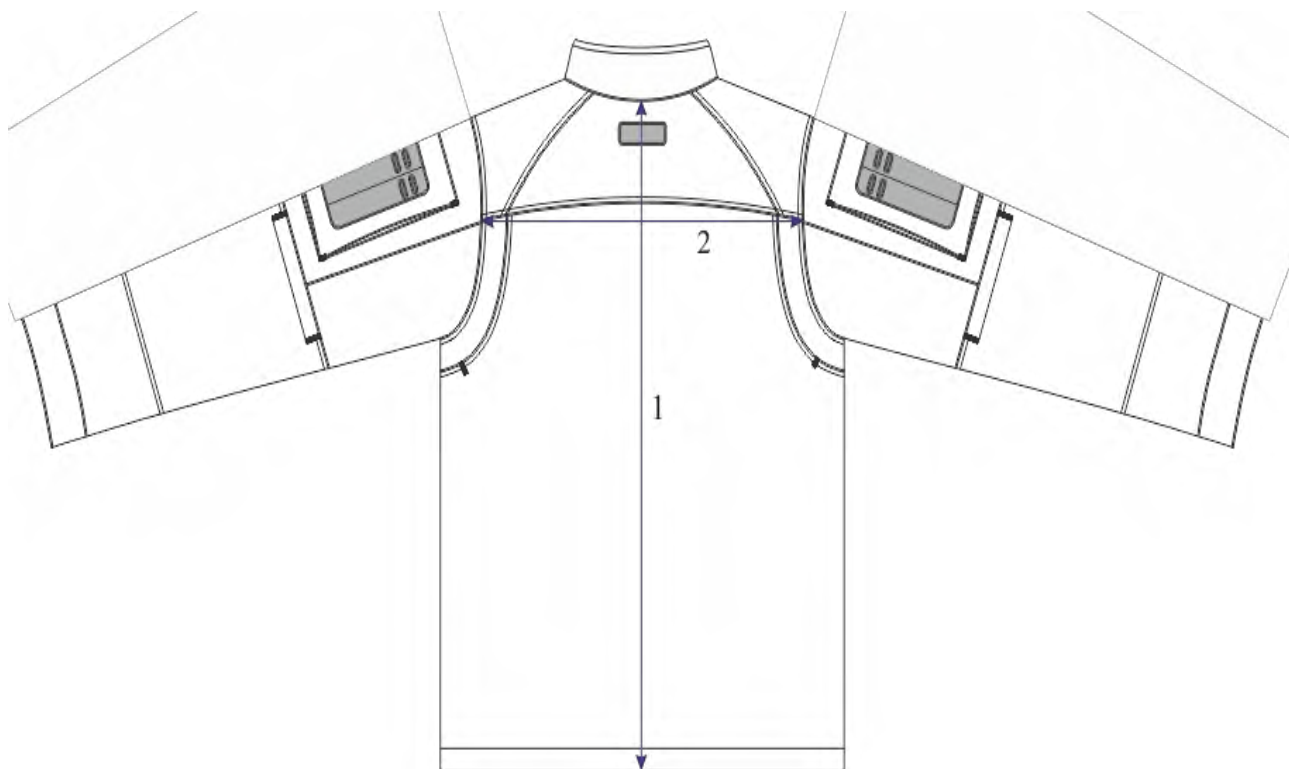
Рисунок ДЗ.2. – Позначення лінійних вимірів предмета 1 (вид ззаду)
