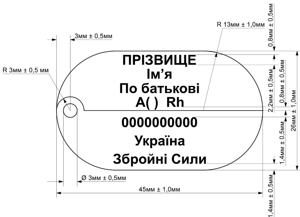
Рисунок 6 Лінійні розміри предмета
